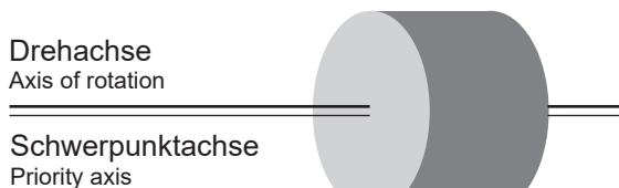
Statische Unwucht Static unbalance
